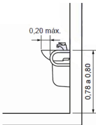
Figura 21 - Vista lateral de instalação de barras laterais horizontais ao lavatório
