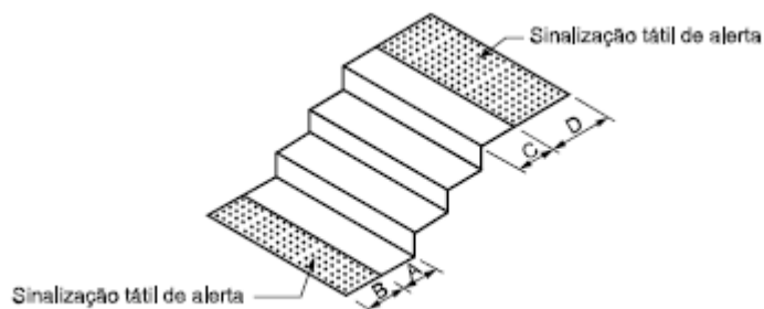
Figura 11 - Escada fixa
