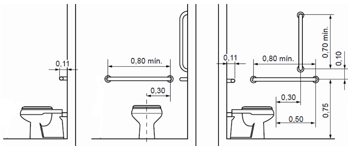
Figura 19 - Posicionamento e dimensões mínimas das barras de apoio
