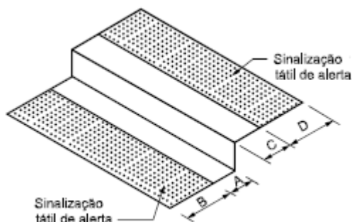
Figura 12 - Degrau isolado
