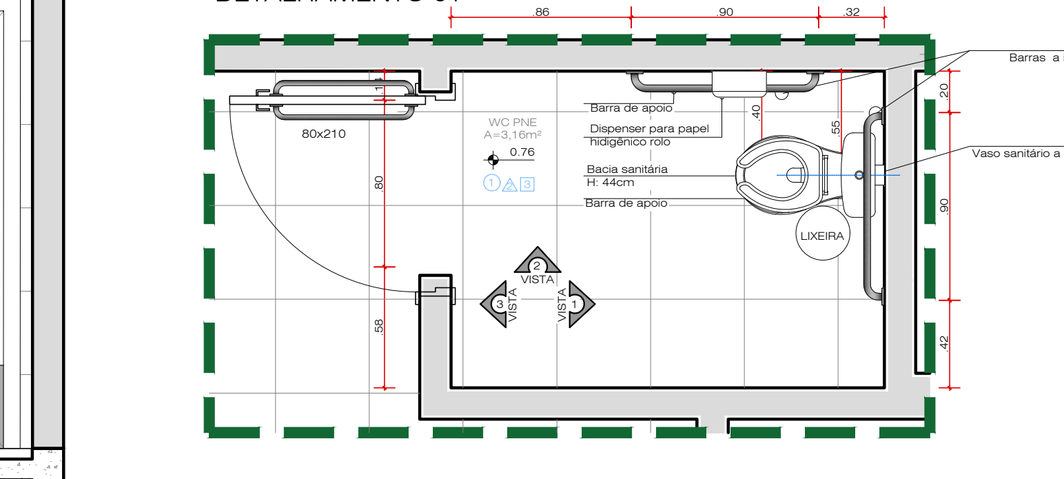
LAYOUT A CONSTRUIR
