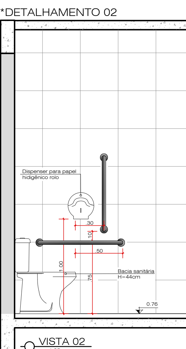
VISTA 02
