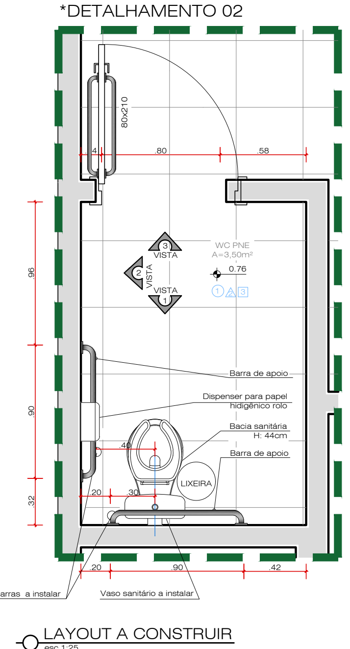
LAYOUT A CONSTRUIR
