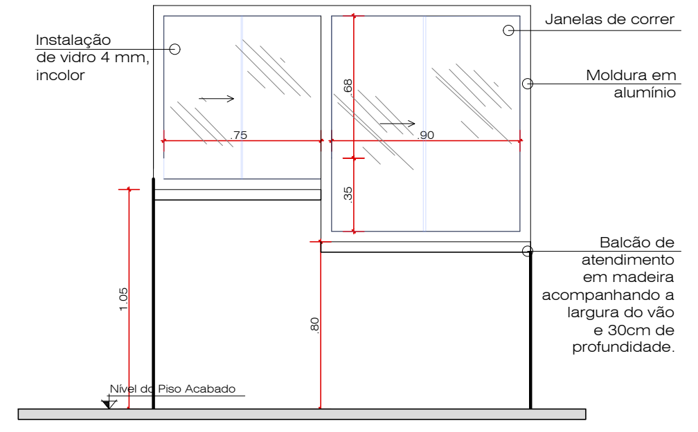
Detalhamento Guichê de Atendimento
