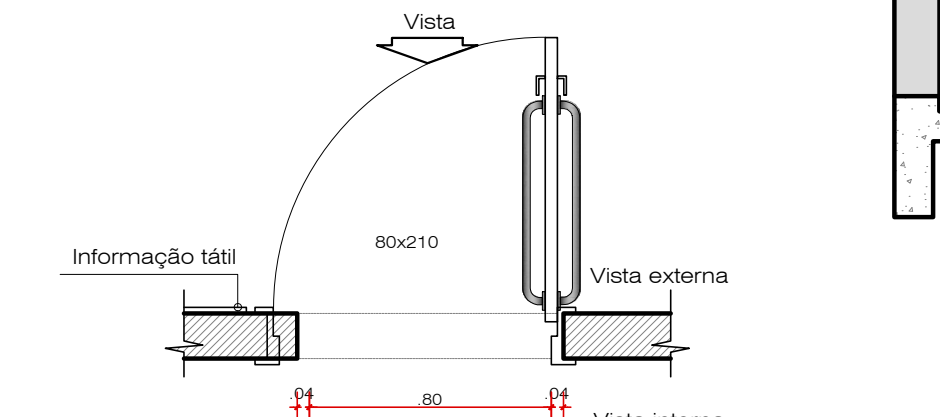
Planta Baixa
