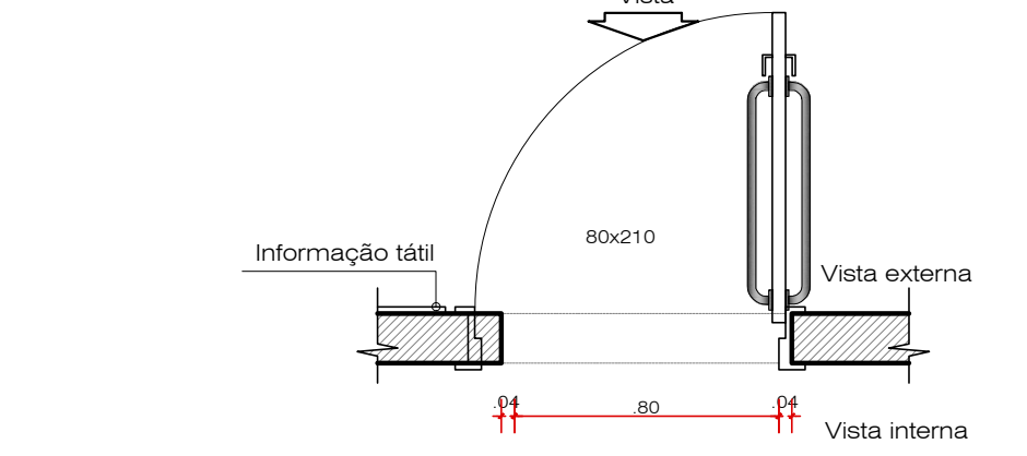
Planta Baixa
