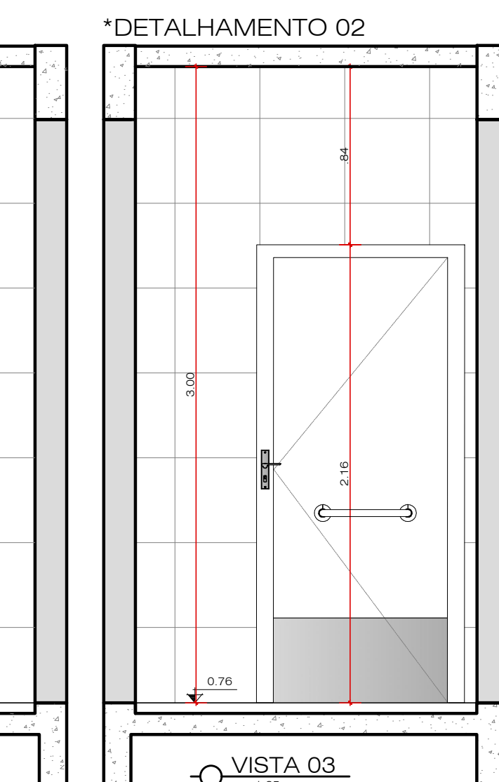
VISTA 03
