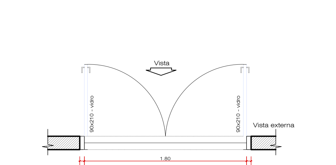
Planta Baixa
