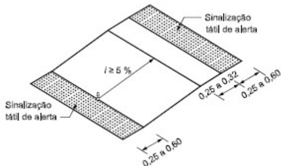
Figura 10 - Rampas fixas i superior a 5%
