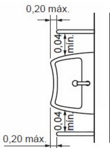
Figura 17 - Planta baixa instalação de barras laterais horizontais ao lavatório
