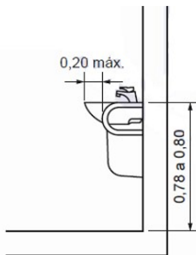
Figura 18 - Vista lateral de instalação de barras laterais horizontais ao lavatório
