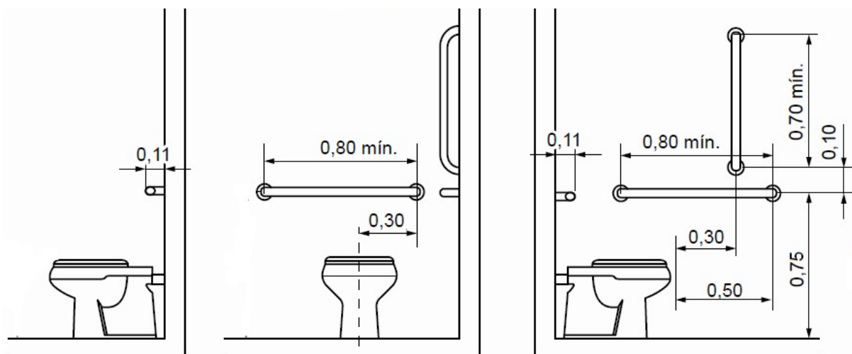
Figura 16 - Posicionamento e dimensões mínimas das barras de apoio
