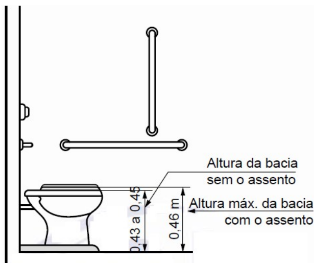
Figura 11 - Altura da bacia – Vista lateral
