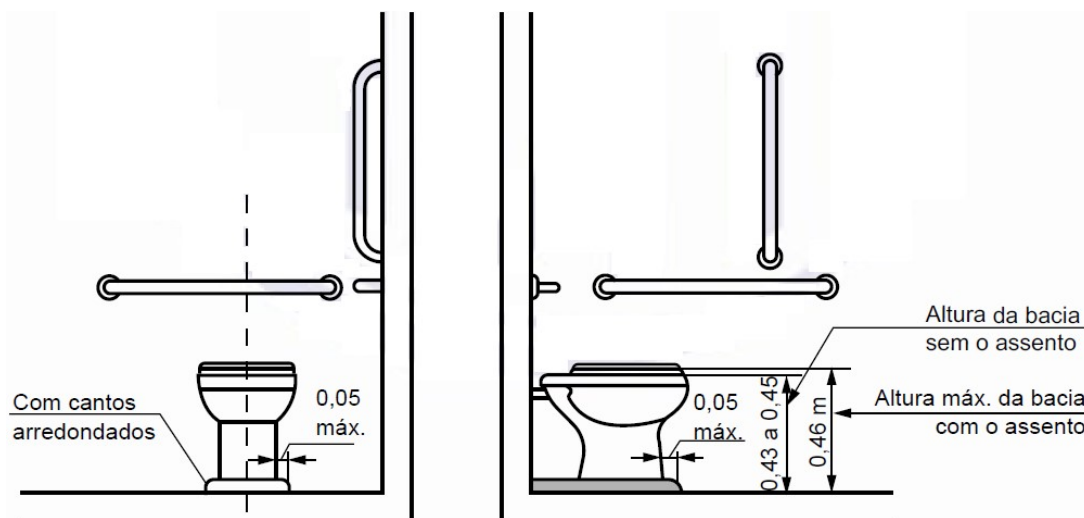
Figura 12 - Vistas frontal e lateral esquerda (bacia instalada sobre sóculo de concreto)
