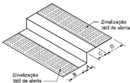
Figura 9 - Degrau isolado
