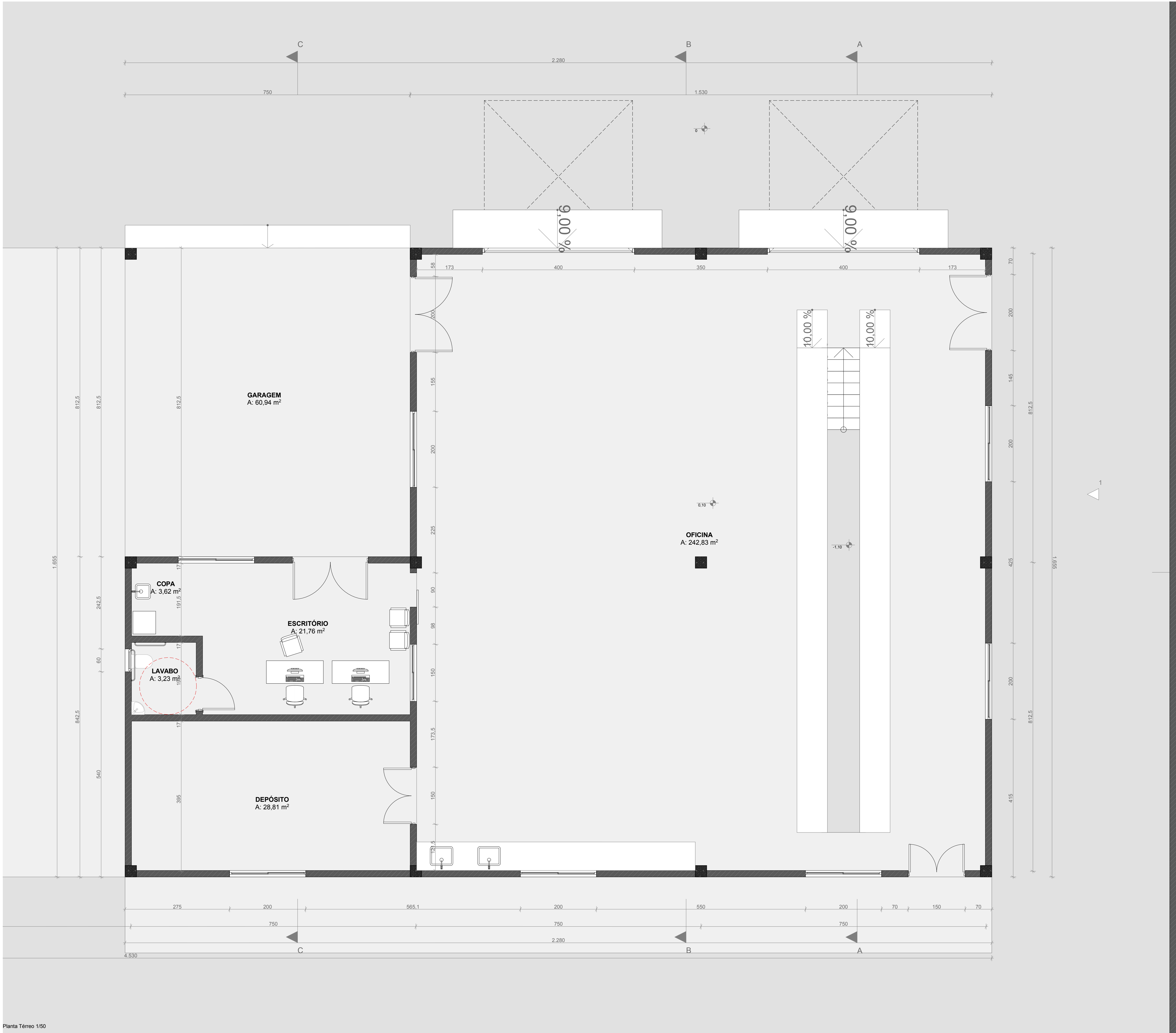
Planta Térreo 1/50
