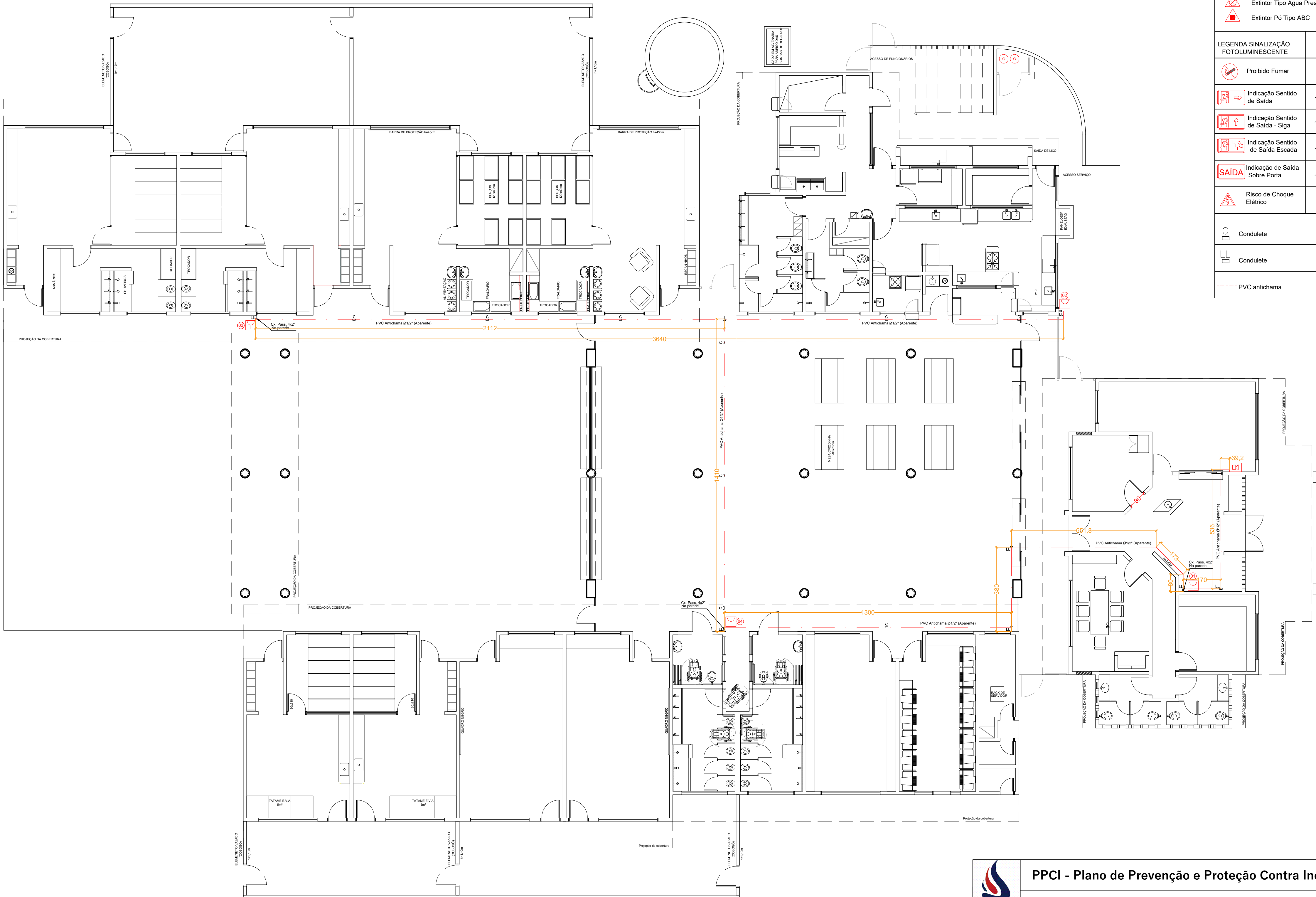
PLANTA BAIXA - PAVIMENTO TÉRREO Esc 1:100
