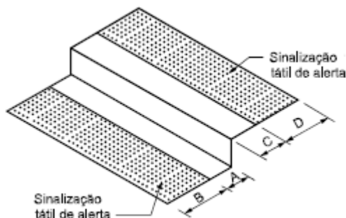
Figura 9 - Degrau isolado
