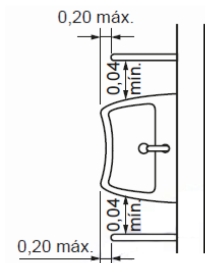
Figura 17 - Planta baixa instalação de barras laterais horizontais ao lavatório
