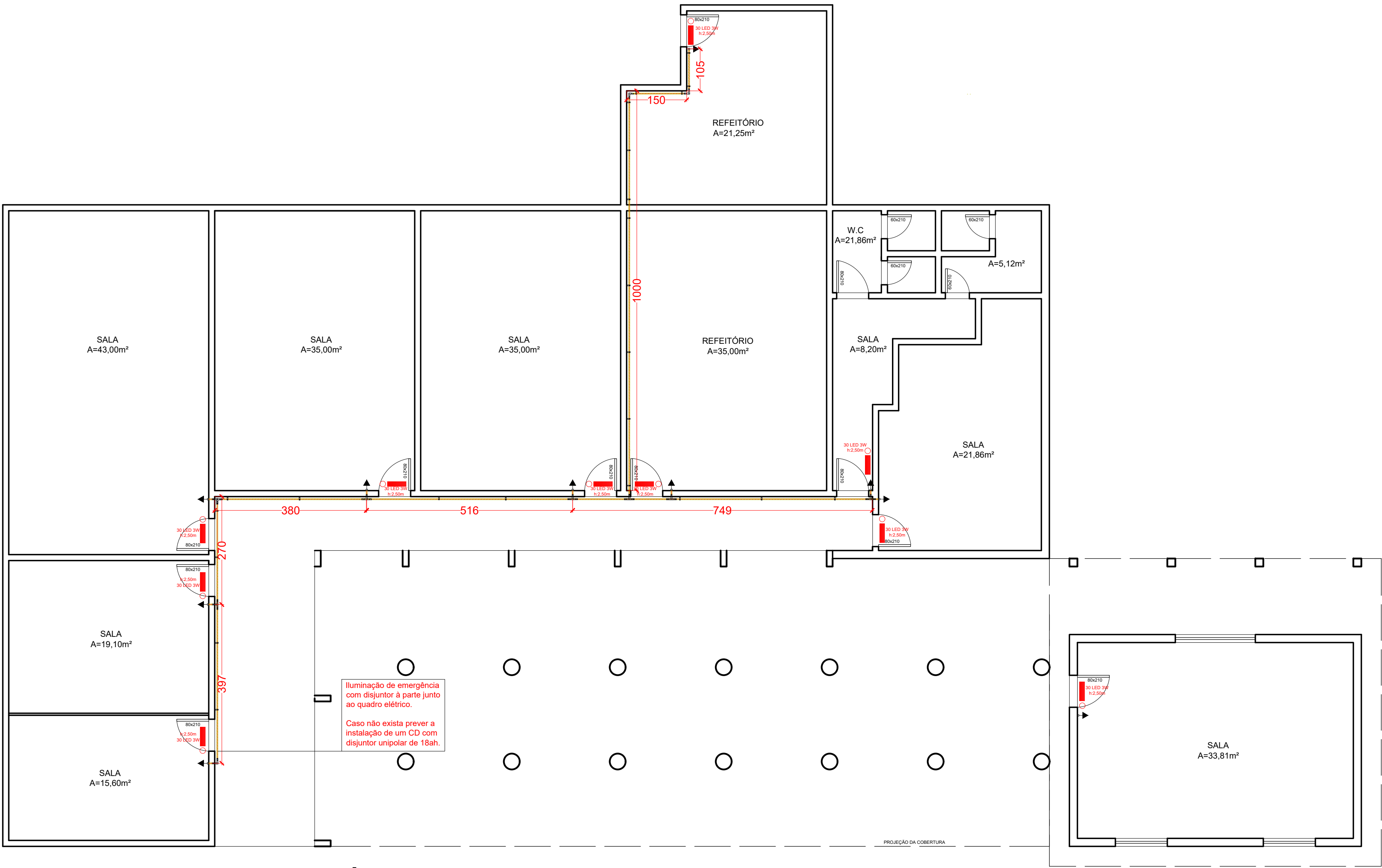
PLANTA BAIXA PAV. TÉRREO Esc 1:75
