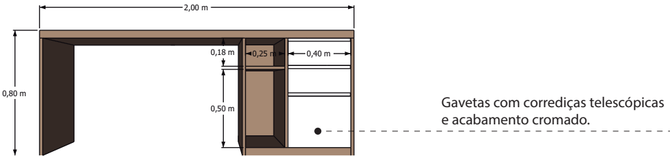
Vista Fundos
