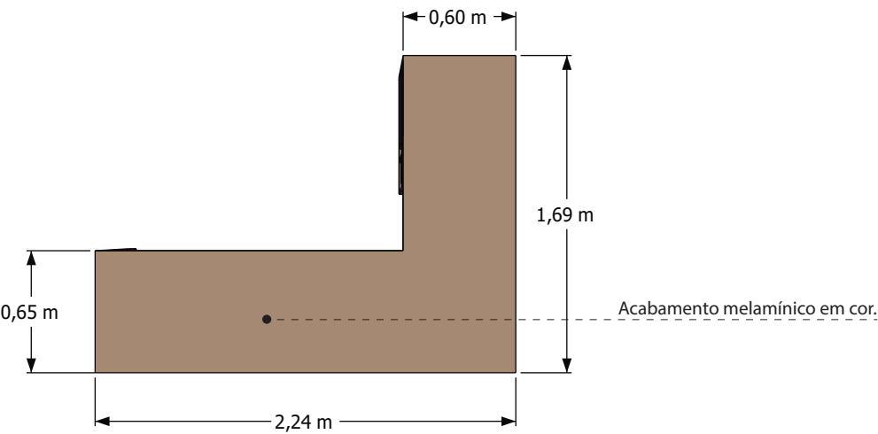
Vista Superior
