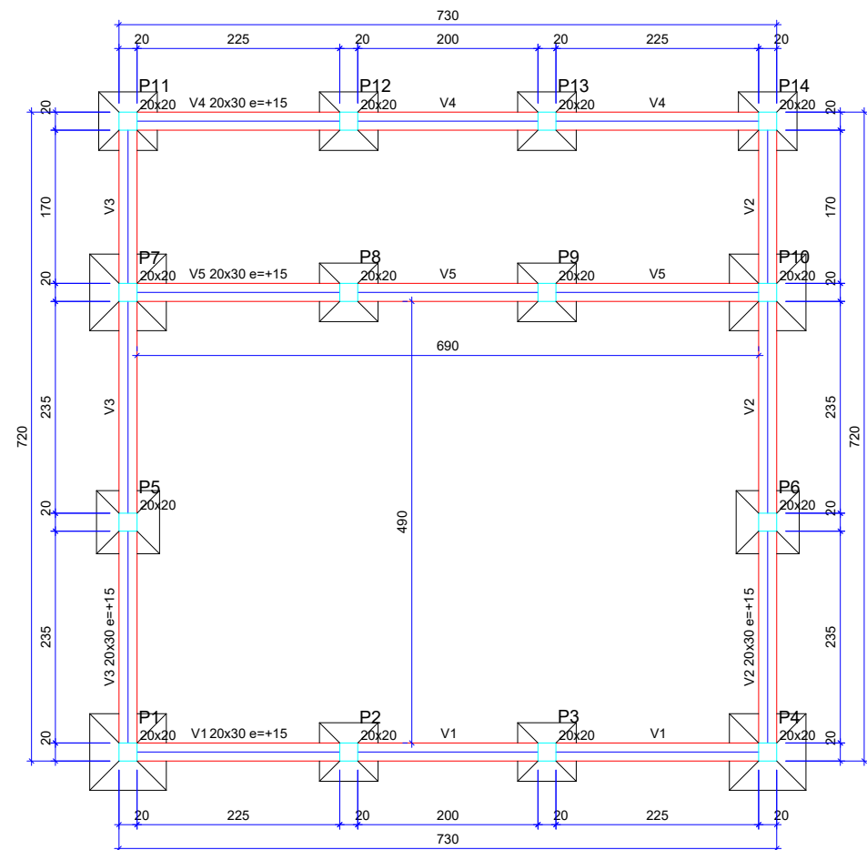
PLANTA DE FORMA BALDRAME
