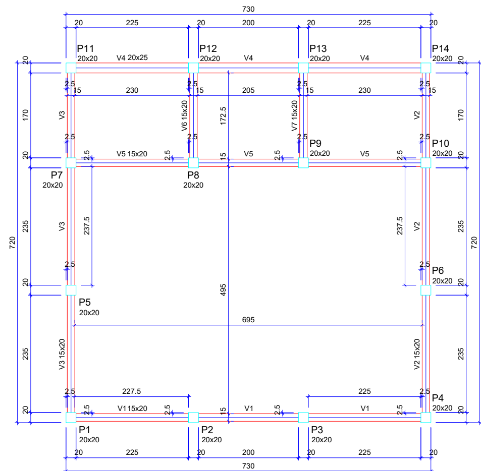
PLANTA DE FORMA VIGAS
